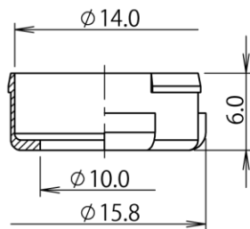
断面図 A-A
