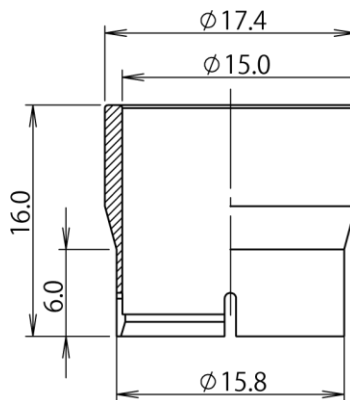
断面図 B-B
